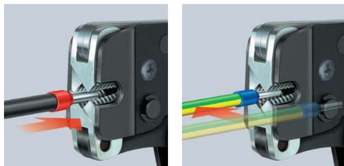
Čelní zavádění dutinek např. ve skříňových rozvaděčích
