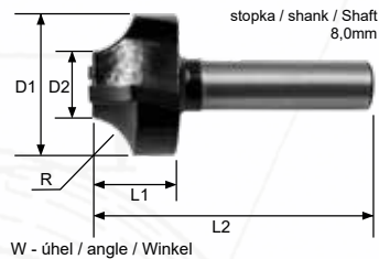
W - úhel / angle / Winkel
